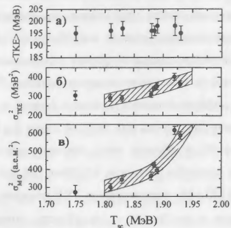
Рис.3. \langle TKE \rangle , \sigma_{TKE}^2 и (\sigma_M^2)_G для реакции ^{48}\text{Ca} + ^{208}\text{Pb} как функции температуры ядра в точке разрыва T_{sc} . Заштрихованные области показывают области изменения дисперсий \sigma_{TKE}^2 и (\sigma_M^2)_G для деления нагретых ядер.
