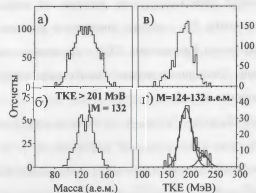
Рис. 4. Слева – массовые распределения фрагментов реакции ^{48}\text{Ca} + ^{208}\text{Pb} при E_{lab} = 211 МэВ для всех фрагментов (а) и для фрагментов с TKE > 201 МэВ (б). Справа – распределения ТКЕ для всех фрагментов (v) и для области симметричных масс M = 124-132 \text{ а.е.м.} (г).
