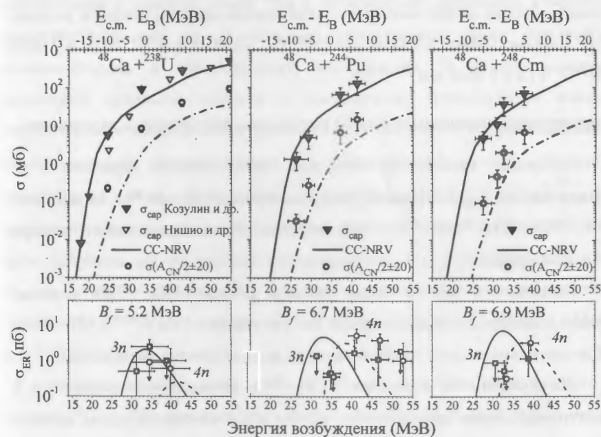
Рис. 9. Сверху: треугольники – сечения делительно-подобных фрагментов в реакциях ^{48}\text{Ca} + ^{238}\text{U} вместе с данными из [15, 17], ^{48}\text{Ca} + ^{244}\text{Pu} , ^{248}\text{Cm} . Сплошные линии – вычисления методом связанных каналов [12], кружки – сечения фрагментов с массами A_{\text{CN}}/2 \pm 20 а.е.м., пунктирные линии с точками – оценки сечений слияния-деления \sigma_{\text{FF}} . Снизу: функции возбуждения для 3n (квадраты) и 4n (круги) испарительных каналов реакции из работы [2]. Сплошными и пунктирными линиями показаны сечения испарительных остатков для 3n и 4n -каналов, вычисленные по полученным в настоящей работе сечениям слияния-деления \sigma_{\text{FF}} .
